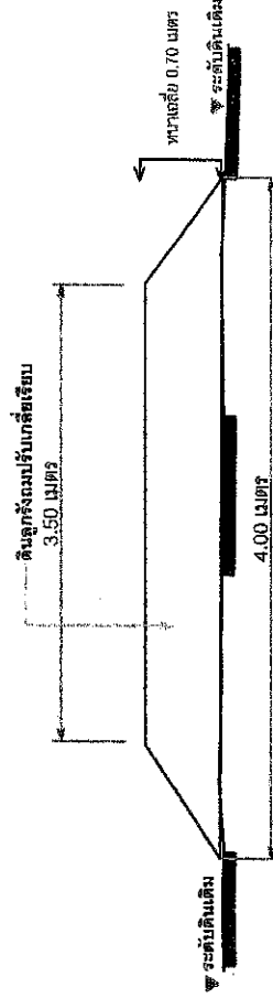
รูปตัด 2-2 NOT TO SCALE
