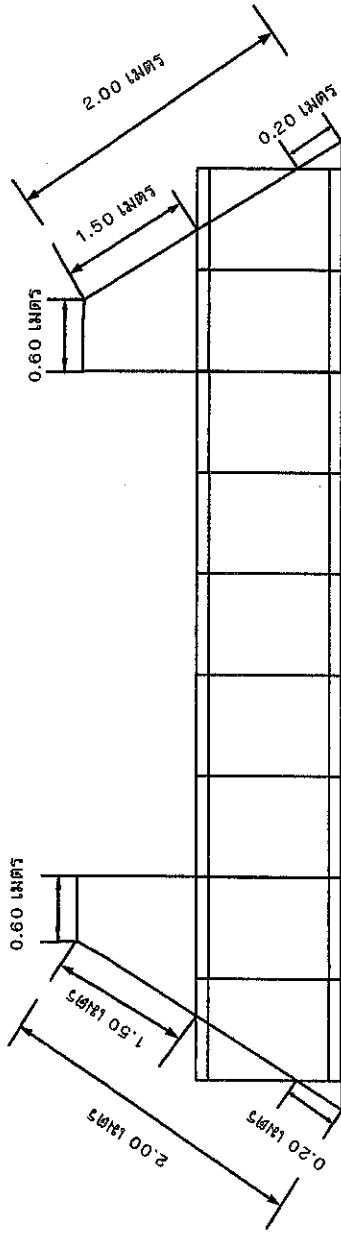
รูปตัดแปดเหลี่ยมคอนกรีต
